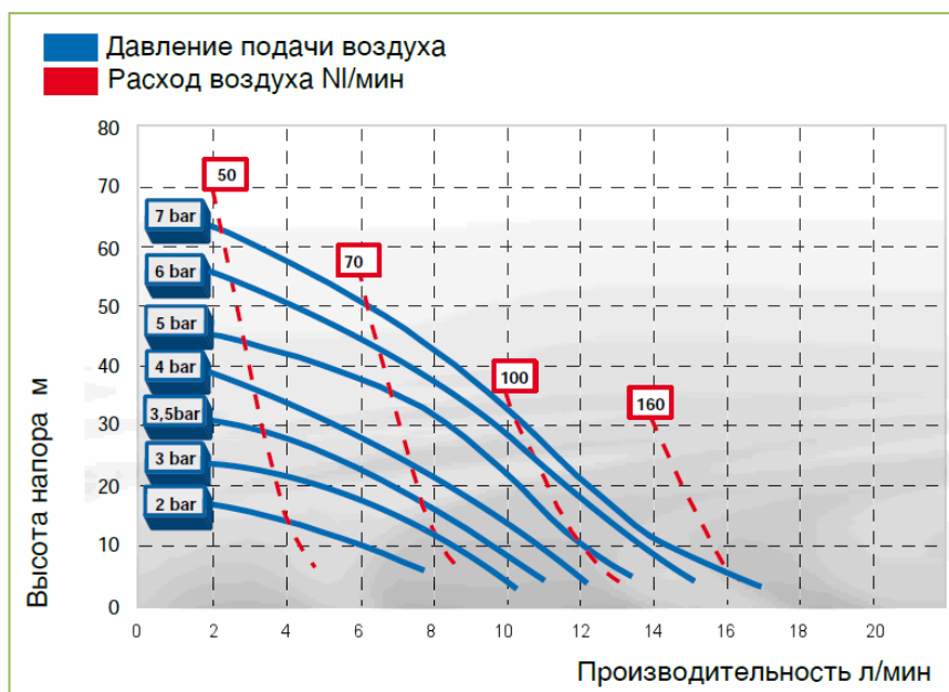
График производительности ABR17
