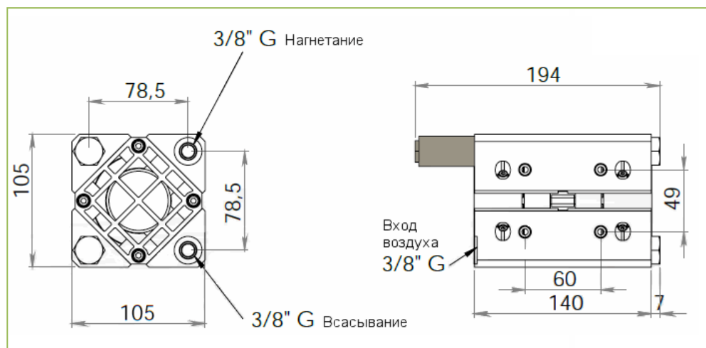
Габаритные размеры ABR17
