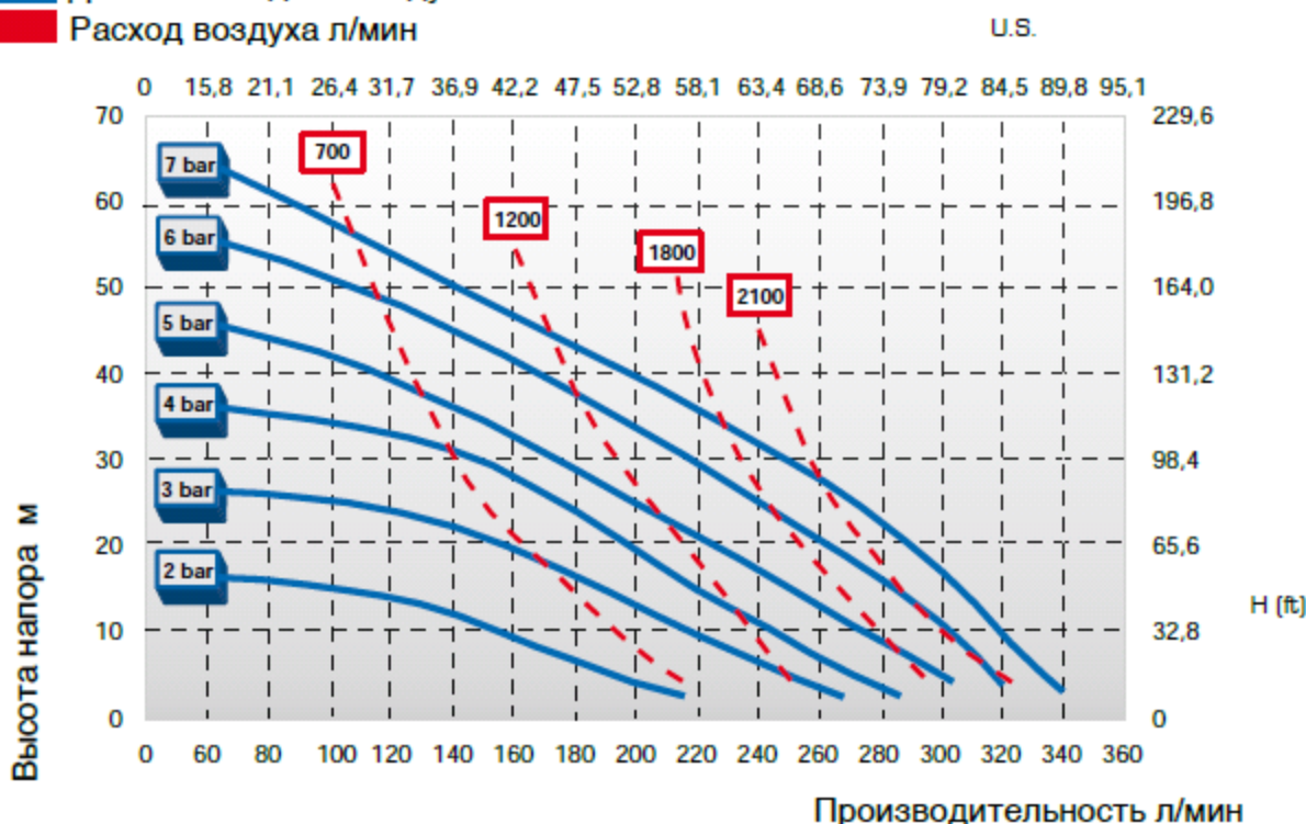
График производительности ABR251
