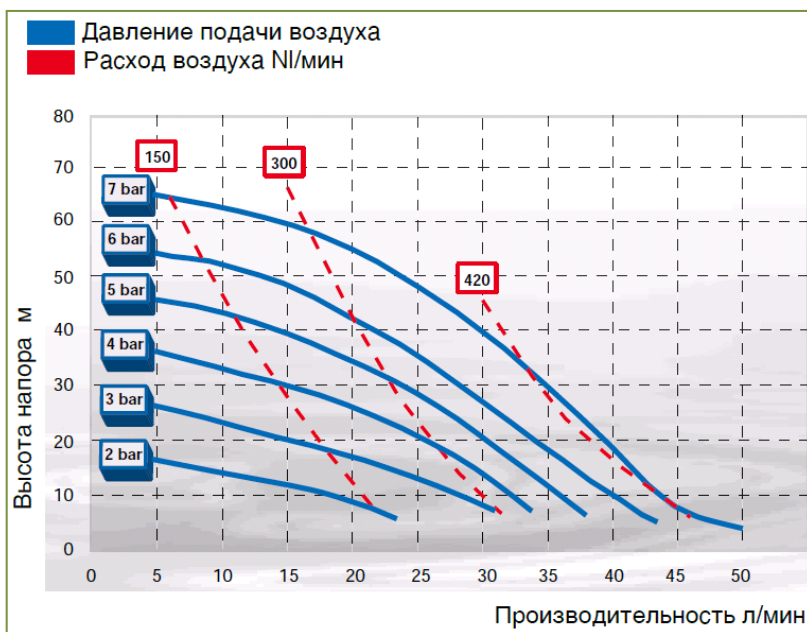
График производительности ABR50
