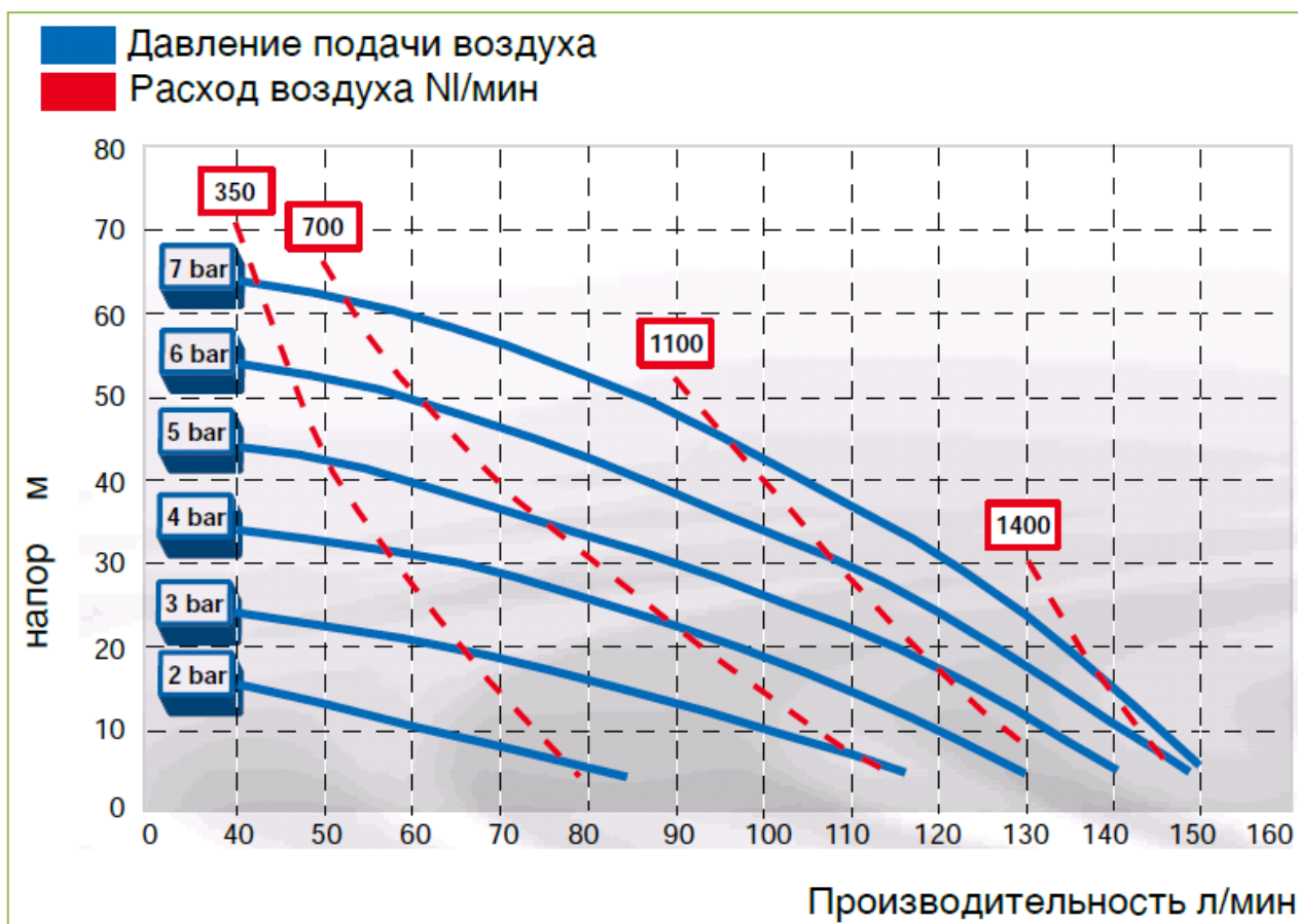
График производительности ABR100
