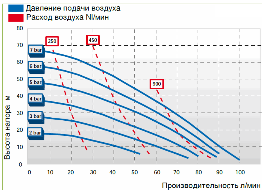
График производительности ABR80-81
