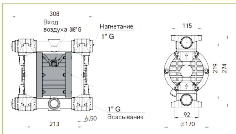
Габаритные размеры ABR80-81
