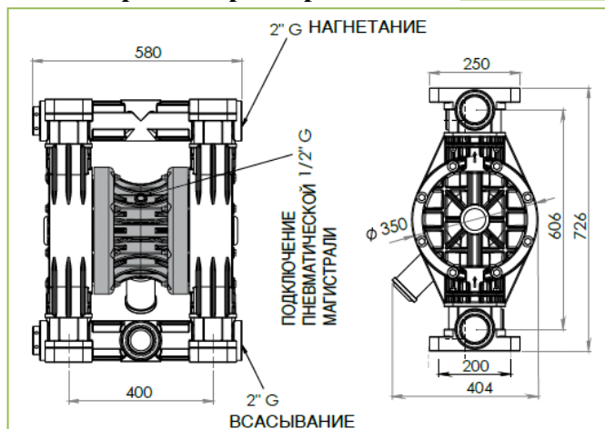
Габаритные размеры ABR502
