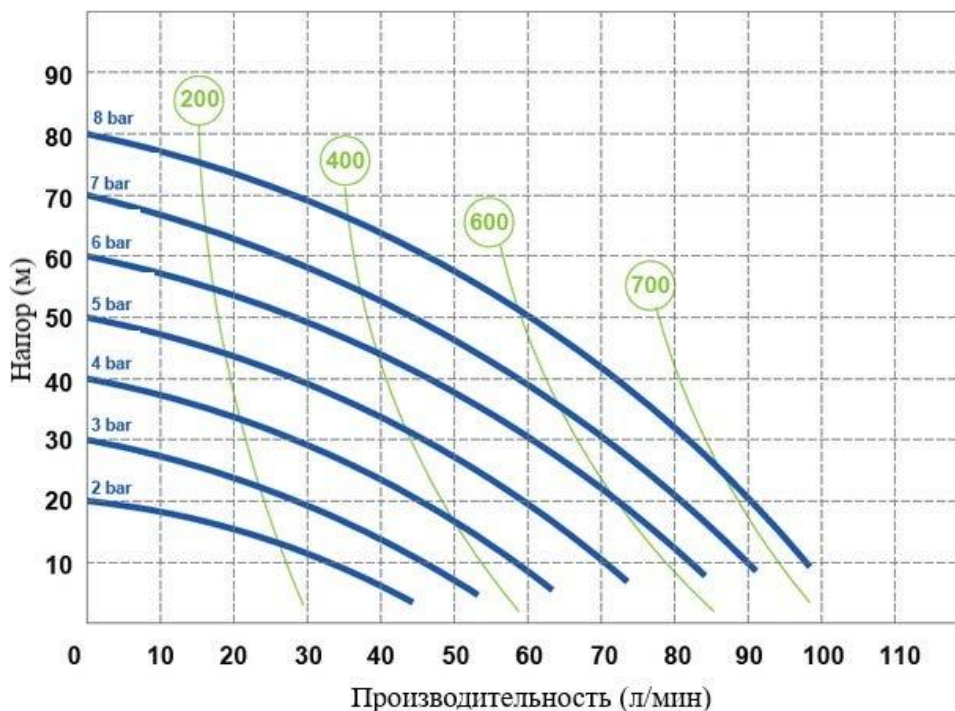
График производительности насосов AFL 90
